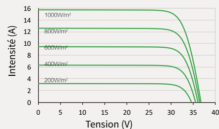
Puissance-Tension (460W)
